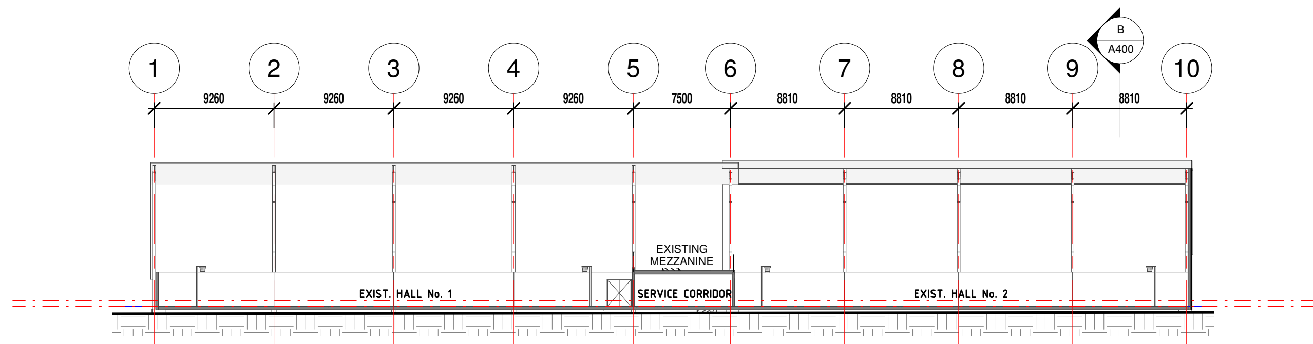
SECTION C 1 : 300
